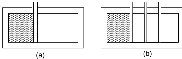
Free expansion
